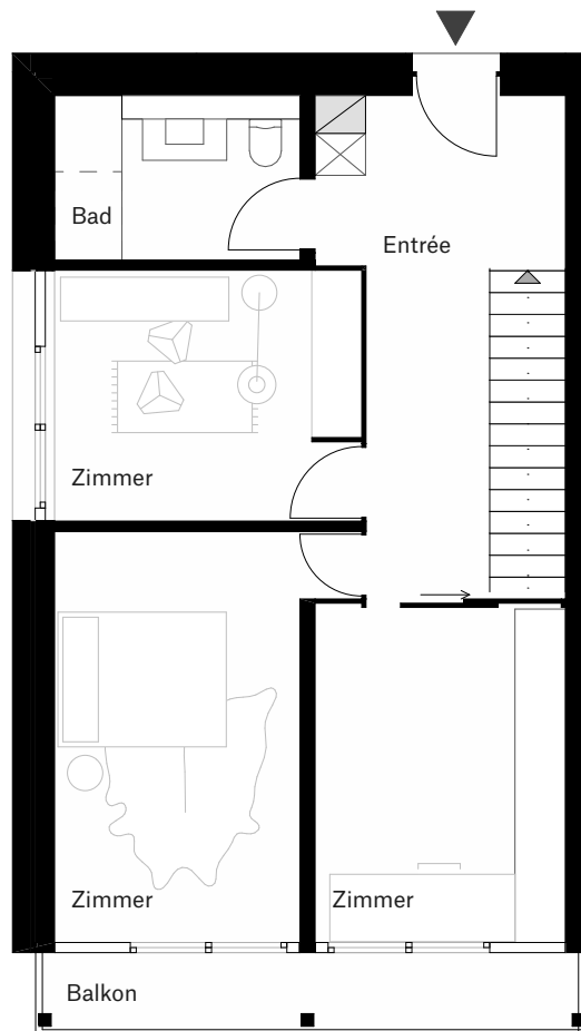
OBERGESCHOSS
