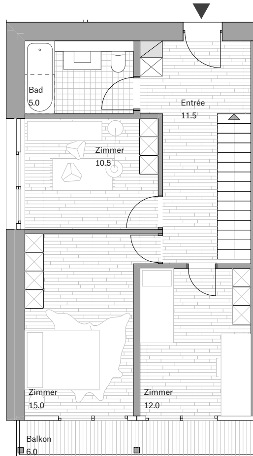
OBERGESCHOSS
